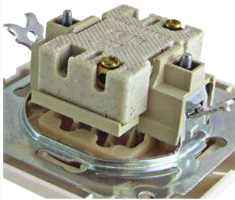
Керамическое основание
