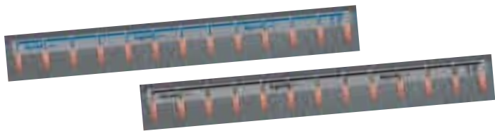
4 049 26 Универсальная гребенчатая шина, фаза + нейтраль черная сторона - фаза, синяя сторона - нейтраль
